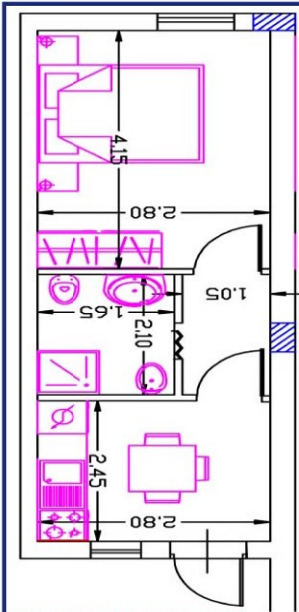
VILLETТА TYPE "A"
