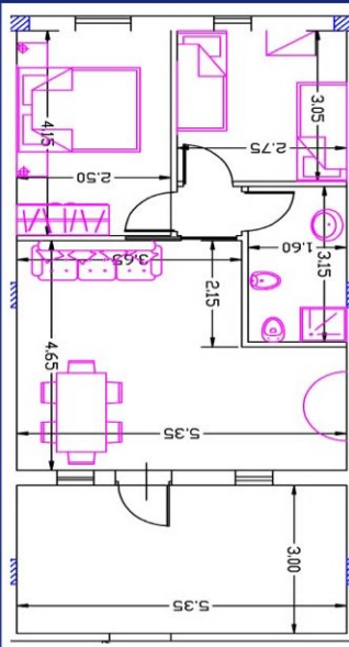
VILLETТА TYPE "C"
